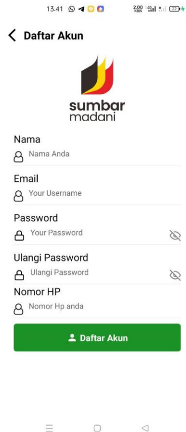
Gambar 9. Halaman Registrasi
