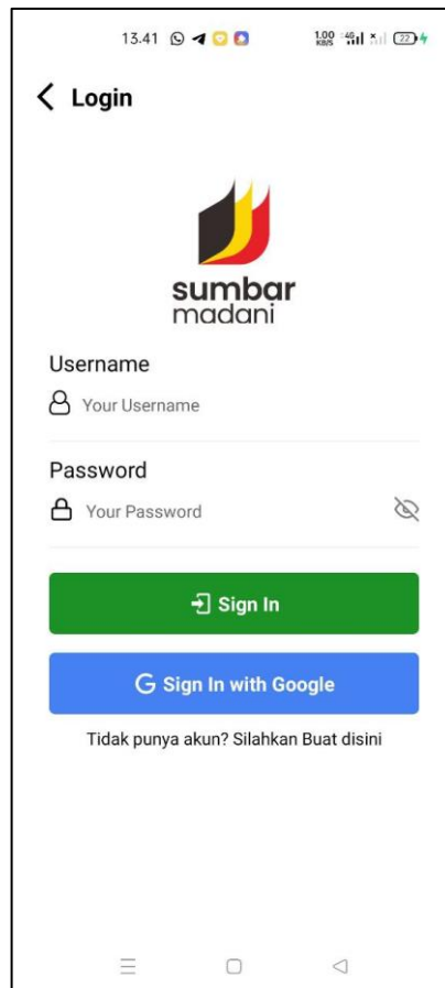
Gambar 10. Halaman Login
