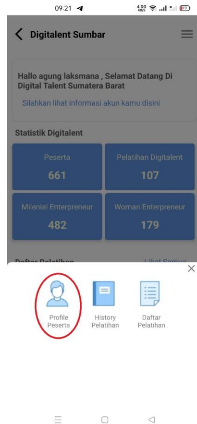
Gambar 13. Menu Profil
