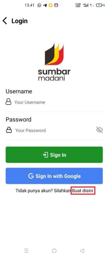
Gambar 8. Pilihan Registrasi
