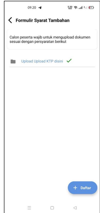
Gambar 14. Syarat Tambahan
